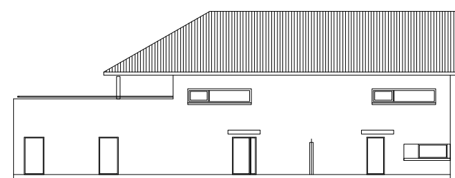
elewacja południowa
