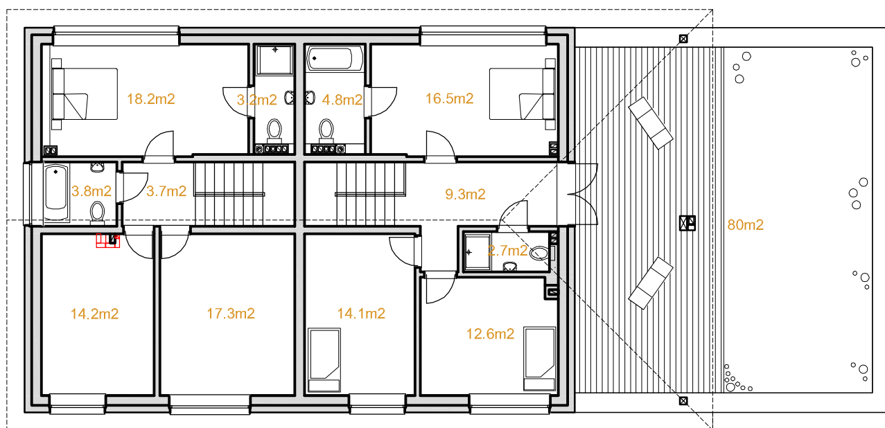
rzut piętra
