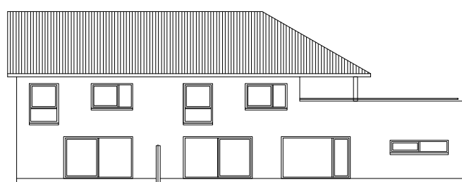
elewacja frontowa
