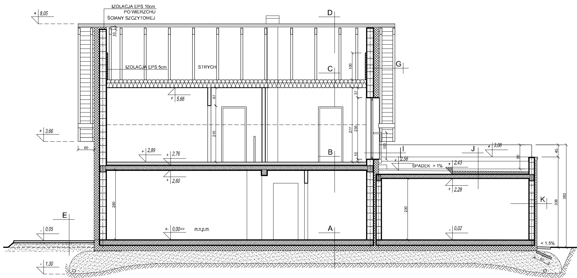
PRZEKRÓJ B-B WARIANT 1. PŁYTA FUNDAMENTOWA
