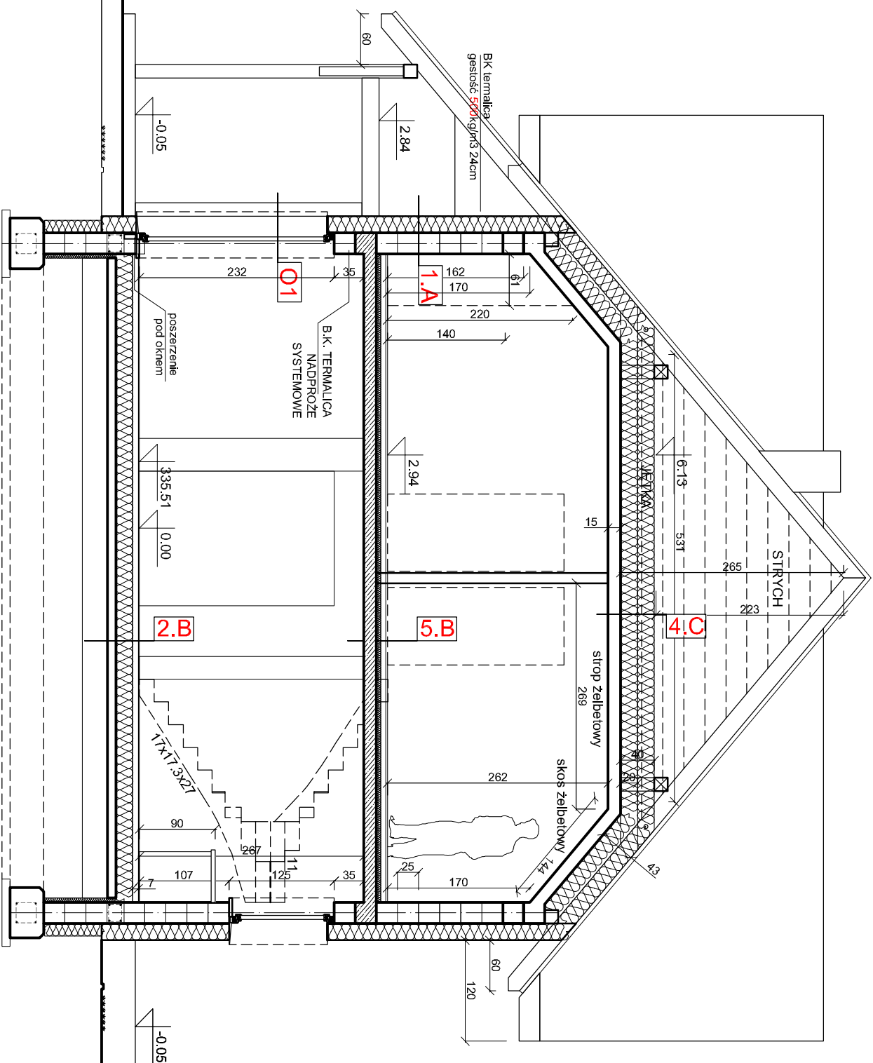
PRZEKRÓJ B-B
