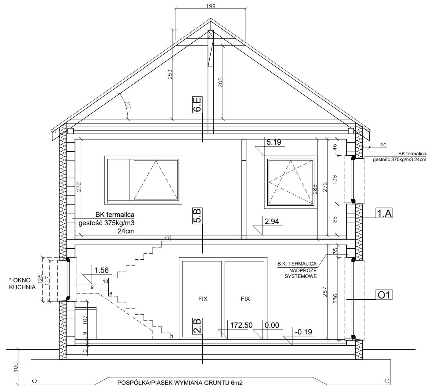
PRZEKRÓJ A-A
