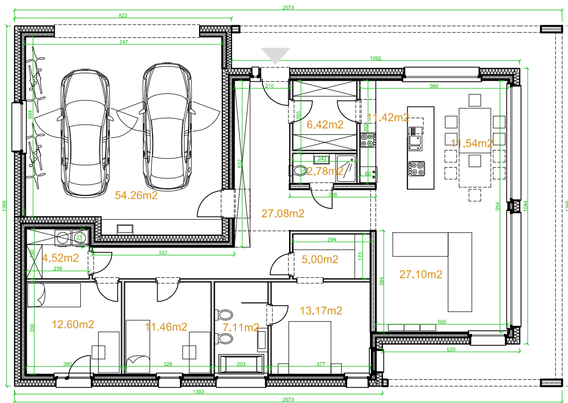
rzut parteru
