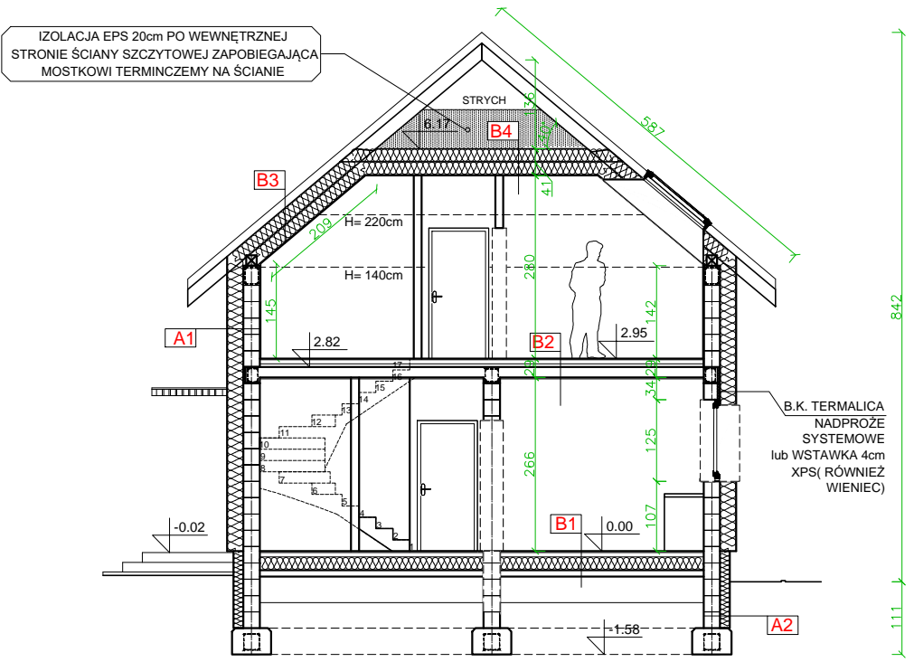
PRZEKRÓJ A-A
