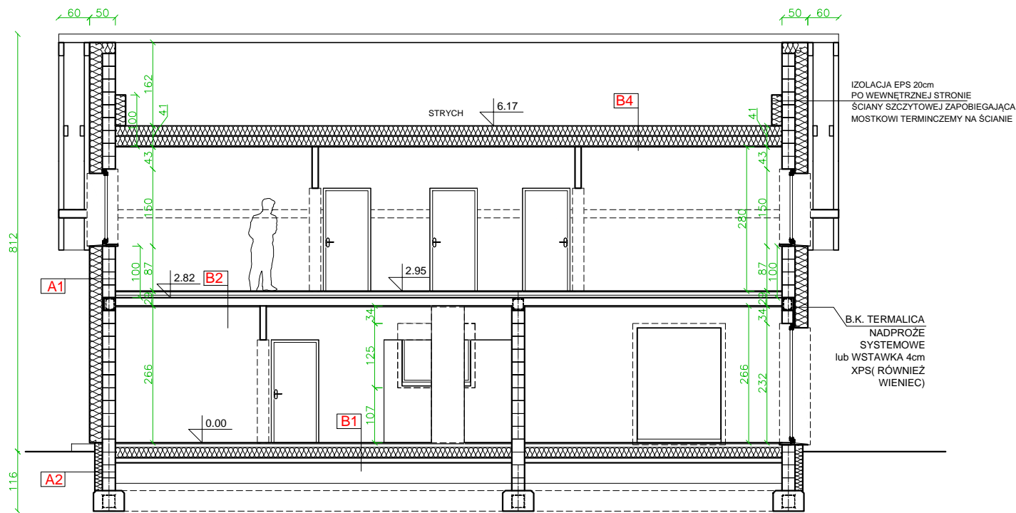
PRZEKRÓJ B-B
