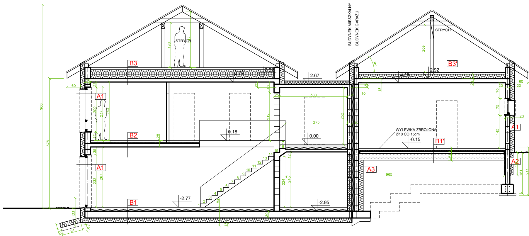
PRZEKRÓJ A-A
