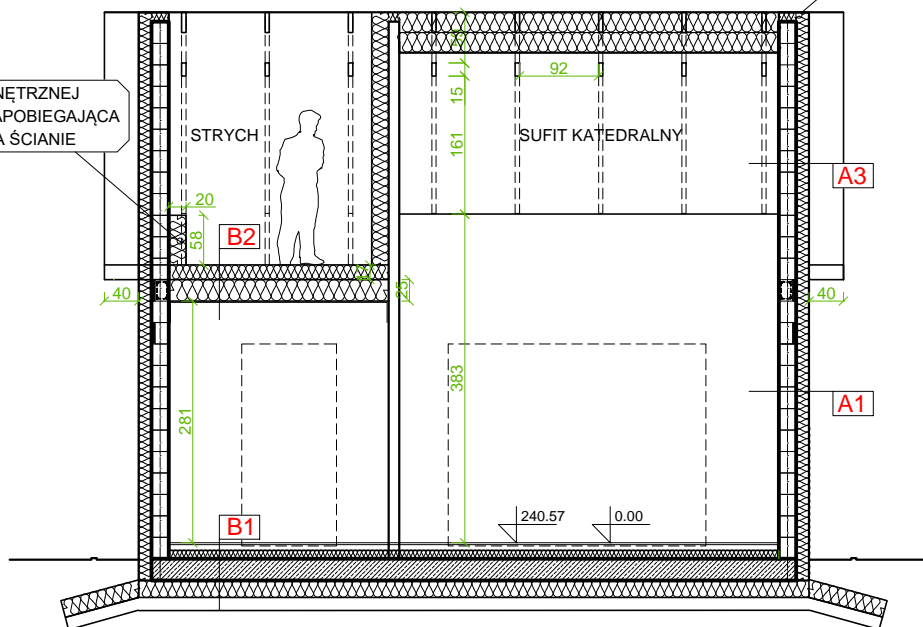
PRZEKRÓJ B-B
