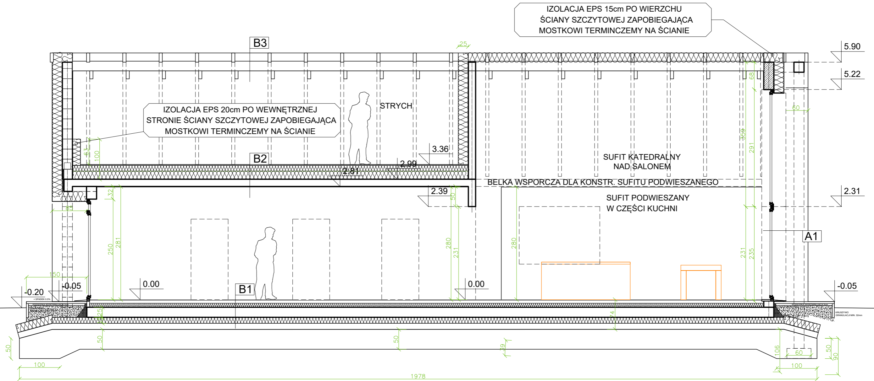
PRZEKRÓJ B-B
