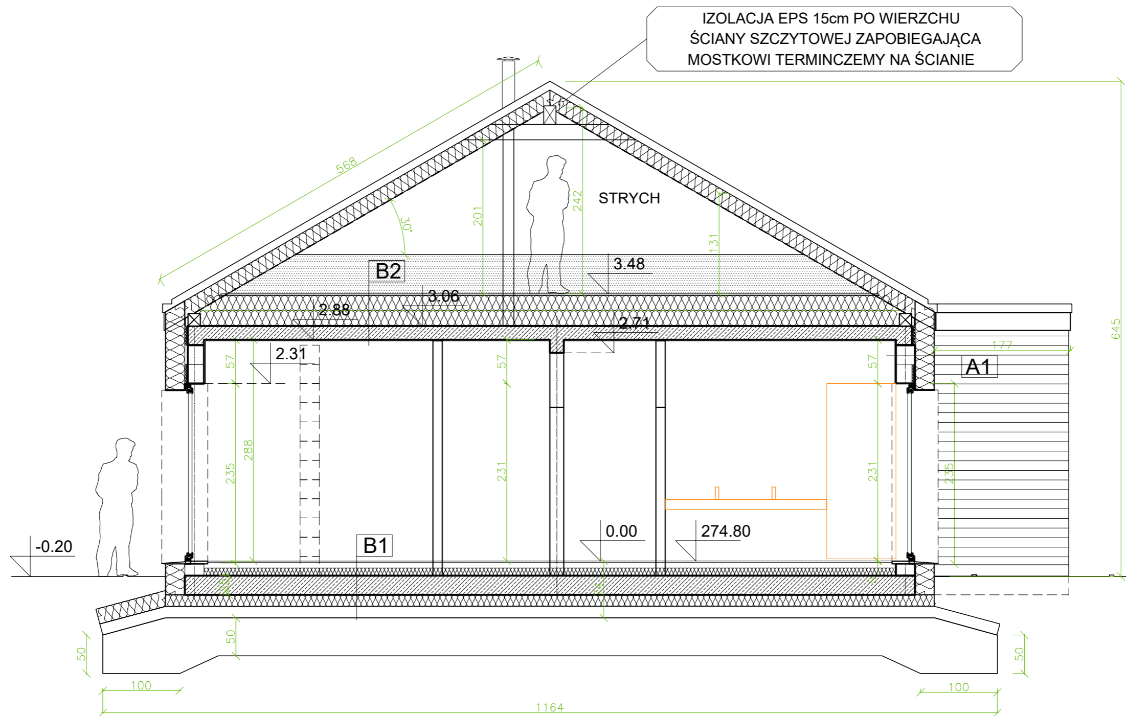
PRZEKRÓJ A-A
