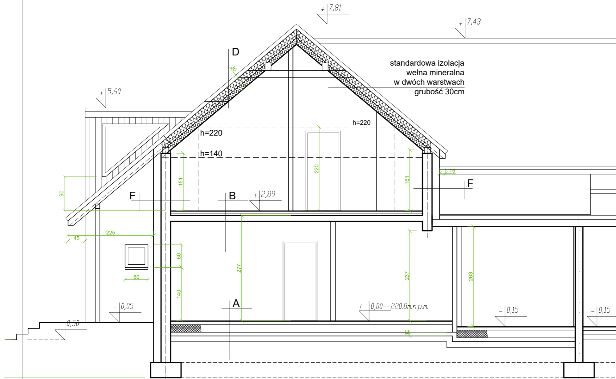
PRZEKRÓJ A-A
