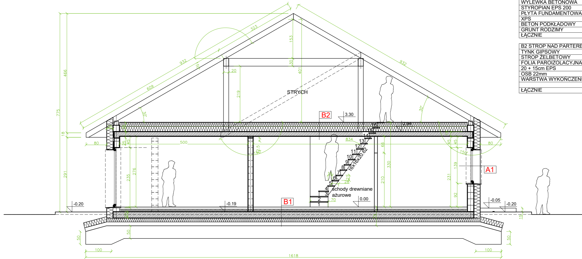
PRZEKRÓJ A-A
