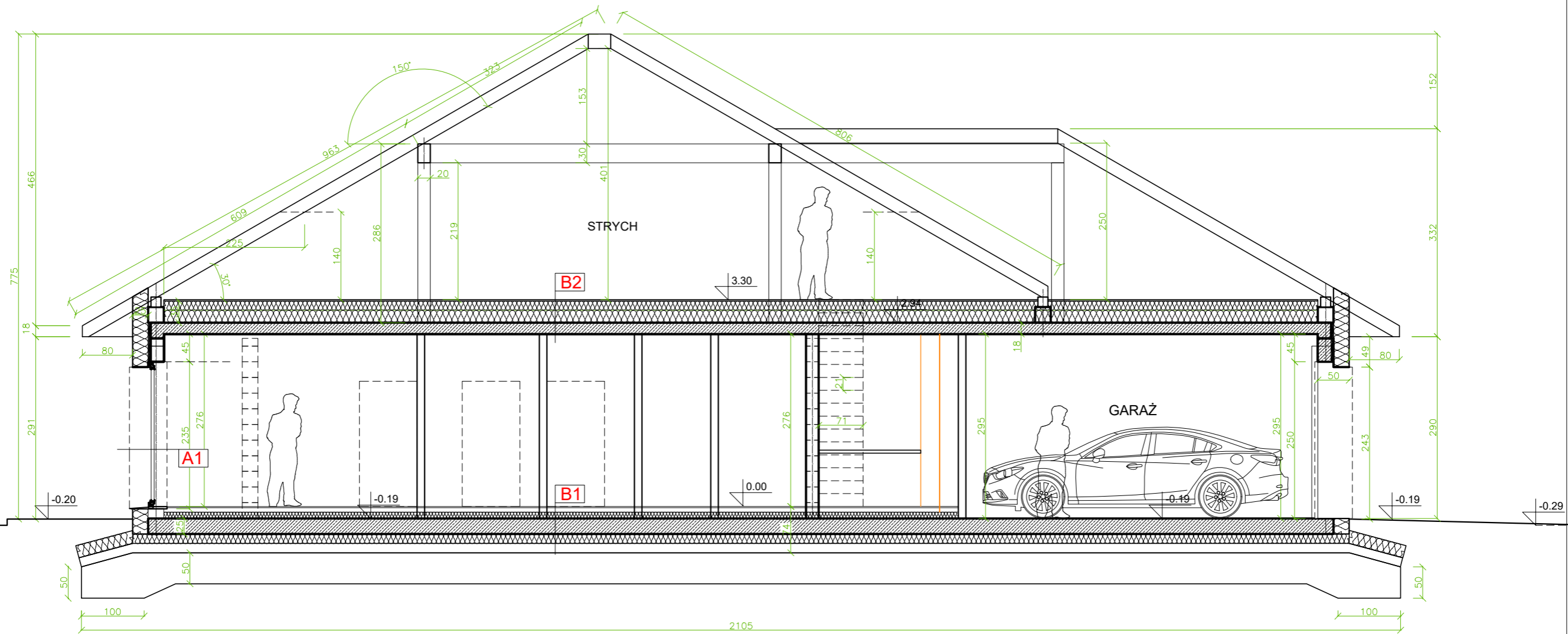
PRZEKRÓJ B-B
