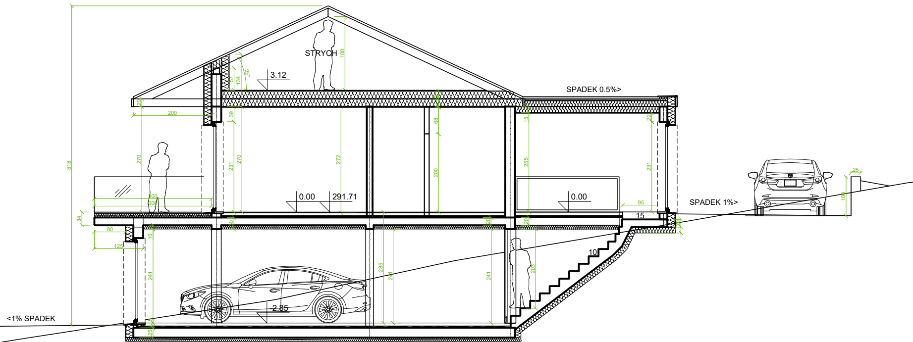
PRZEKRÓJ A-A
