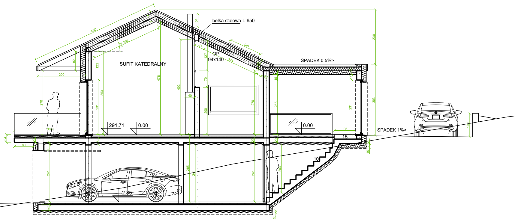
PRZEKRÓJ B-B
